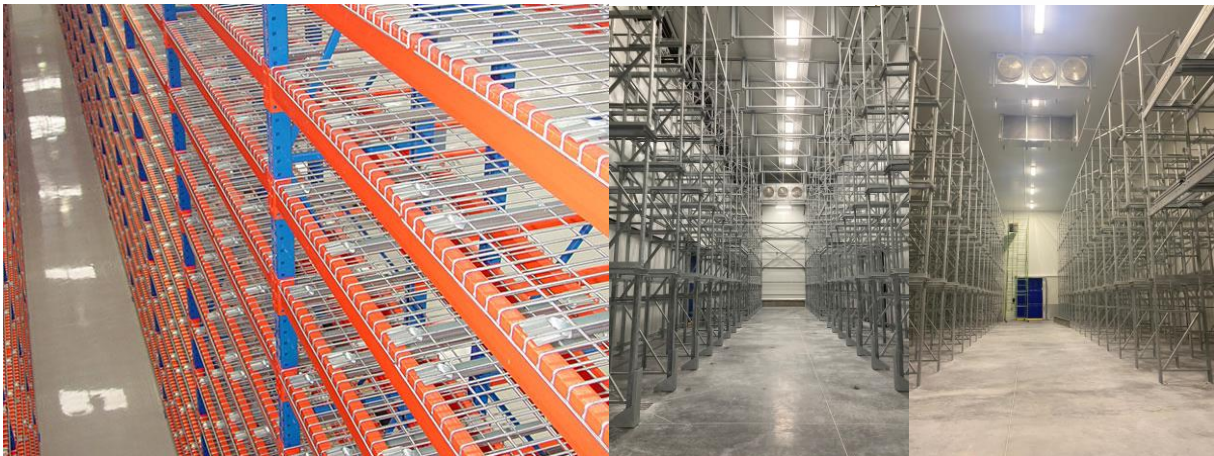
Vigas en naranja y marcos en azul (pintura horneada)
