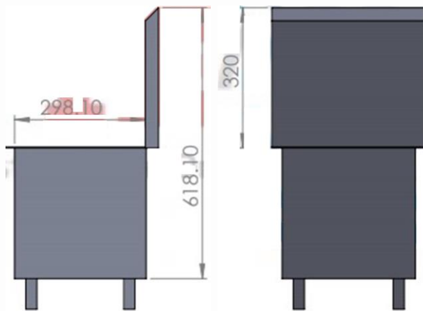
Diagrama de vista lateral del sink
