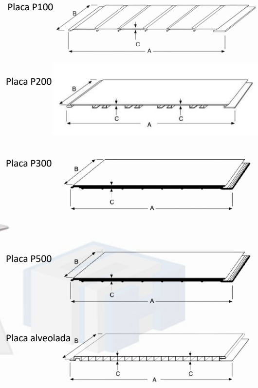
Diagramas de dimensiones de las placas, consultar tabla de abajo.
